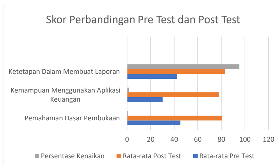
Gambar 1. Grafik Perbandingan Pre Test dan Post Test
